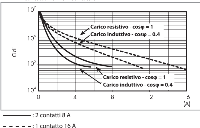
F 38 - Durata elettrica (AC) in funzione della corrente, 1 contatto 16 A e 2 contatti 8 A
