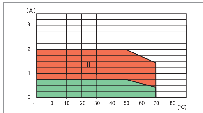
L 34 - Corrente AC di uscita in funzione della temperatura ambiente 38.x1.x.xxx.8240 (solo 38.81/91/21)
