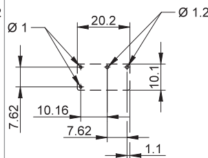
Aanzicht op de aansluitingen
